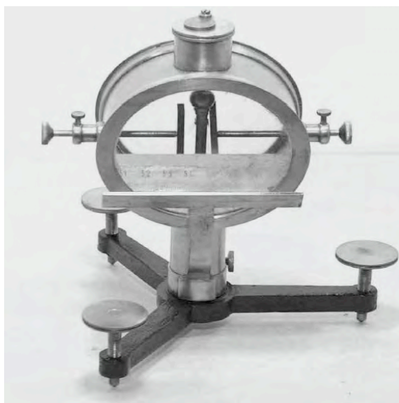
Fig. 3. – Un elettroscopio di Elster e Geitel degli inizi del ventesimo secolo. Questo strumento è composto da un elettroscopio attraverso il quale può essere pompato un flusso d'aria. Per gentilezza del Gabinetto di Fisica dell'Istituto Calasanzio di Empoli.
