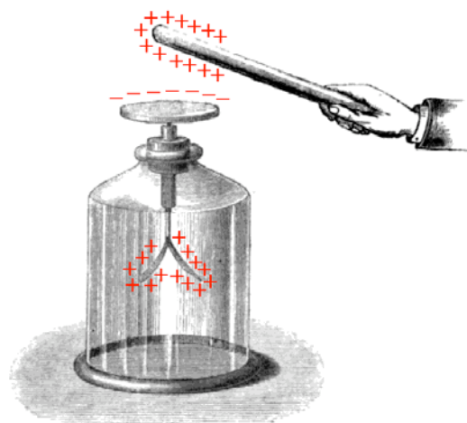
Fig. 2. – Funzionamento schematico dell'elettroscopio.
